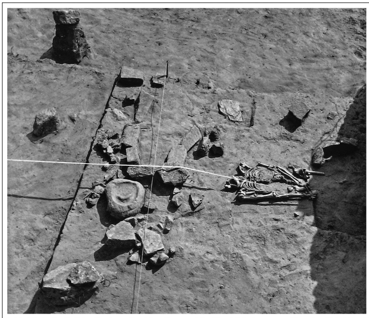
Слика 80. Св. XXXIII, Помрачења Сунца и Месеца; гр. 28
