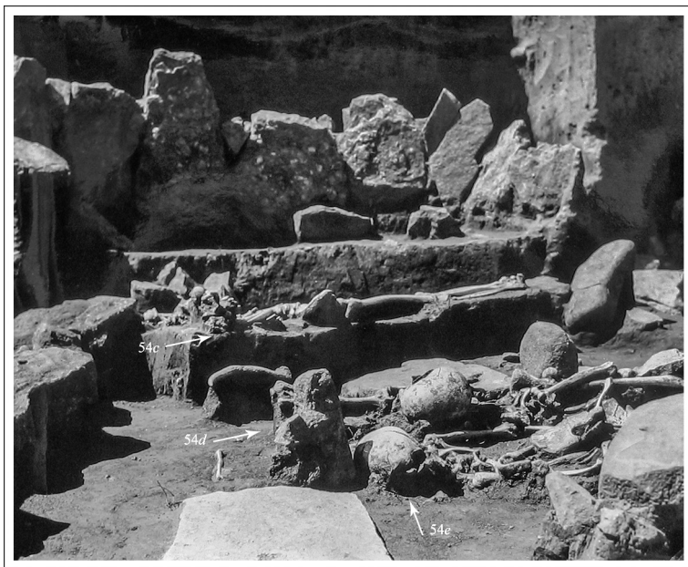
Слика 25. Св. 65/XXXV, Јужна Месечева палата; нивои сахрана у св. 65: гр. 54 с, d, е, са И
