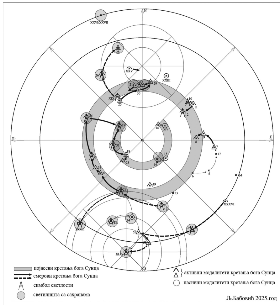
Слика 47. План свет. сфере ноћи, са означеним свет. са сахрањенама
