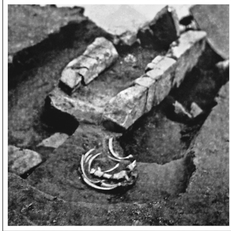
Слика 72. Св. 43, гр. 104
