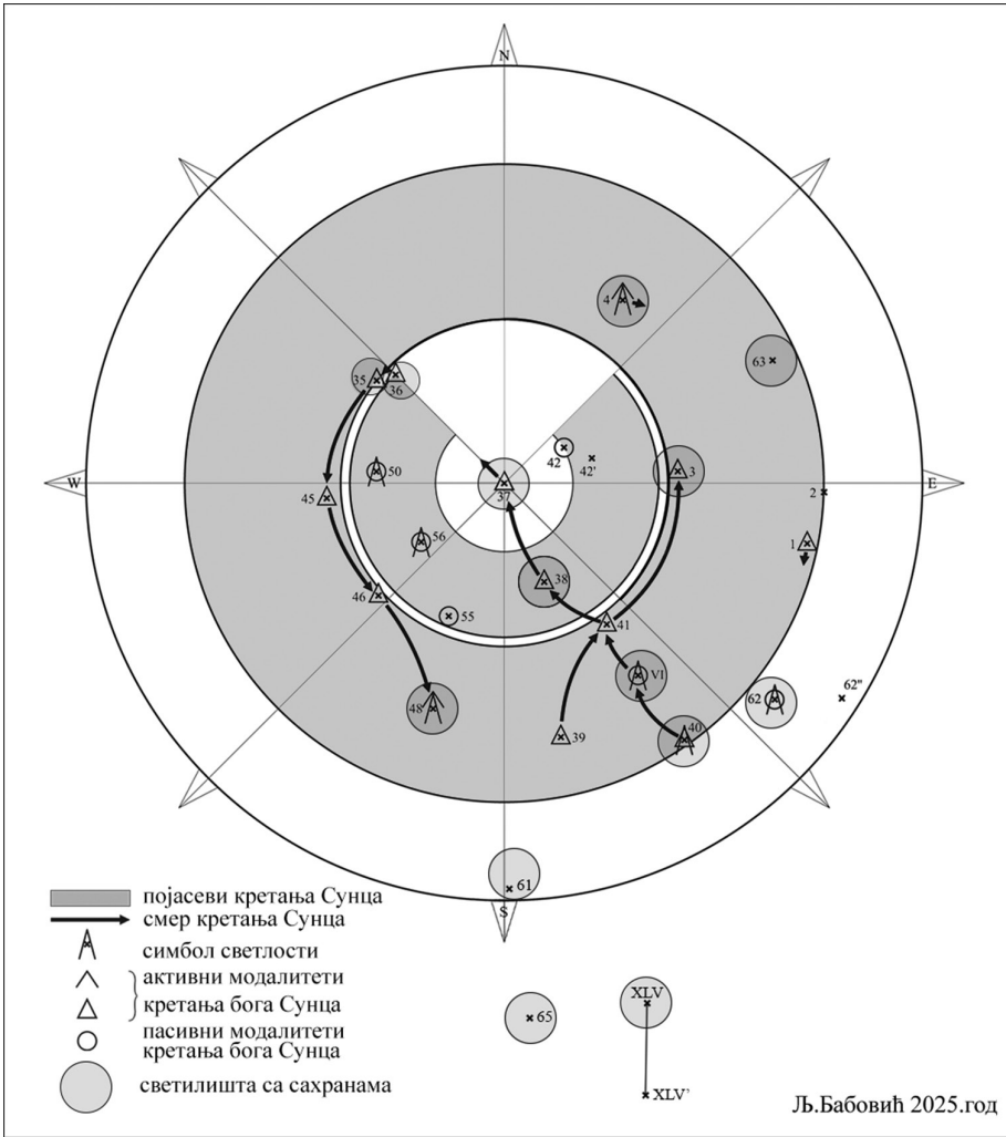
Слика 42. План свет. сфере дана, у односу на зенит, са означеним свет. са сахранама
