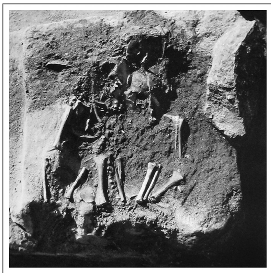
Слика 61. Св. 19, Помрачења Месеца, гр. 103
