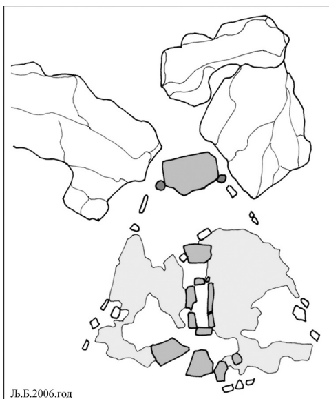
Слика 67. Основа св. 28, Светилиште међу стенама
