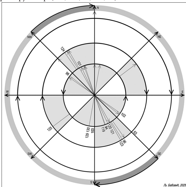
Слика 82. Оријентације скелета новорођенчади, у сфери ноћи
