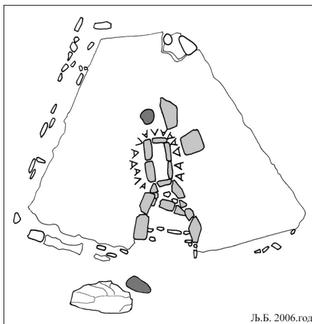
Слика 58. Основа св. 19, Помрачења Месеца
