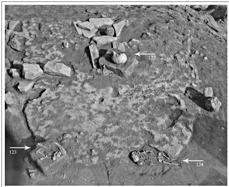
Слика 69. Св. 47;47', Копча сфера, гр. 122,123,124
