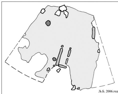
Слика 50. Основа св. 21, Св. Северни Сунчев Обрт
