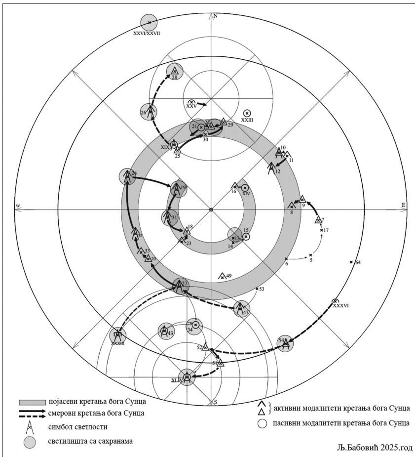
Слика 81. План свет. сфере ноћи, са означеним свет. са сахранама
