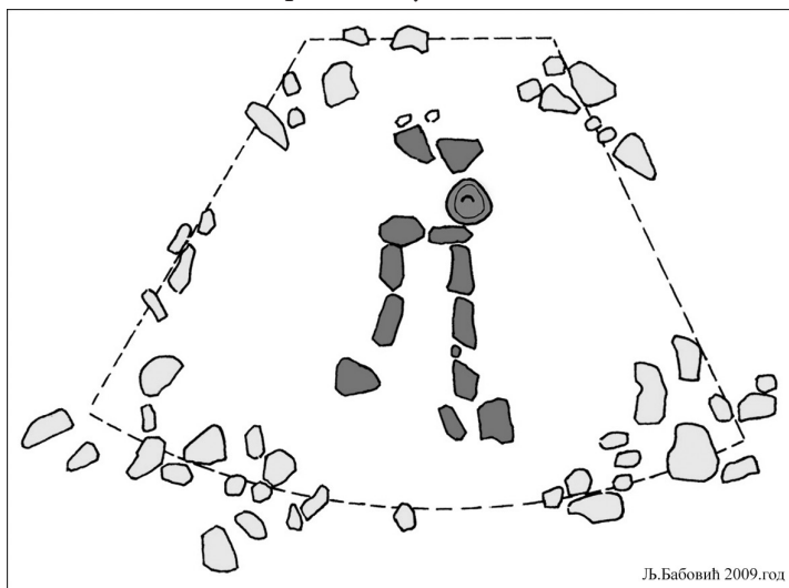
Слика 79. Основа св. XXXIII, Помрачења Сунца и Месеца
