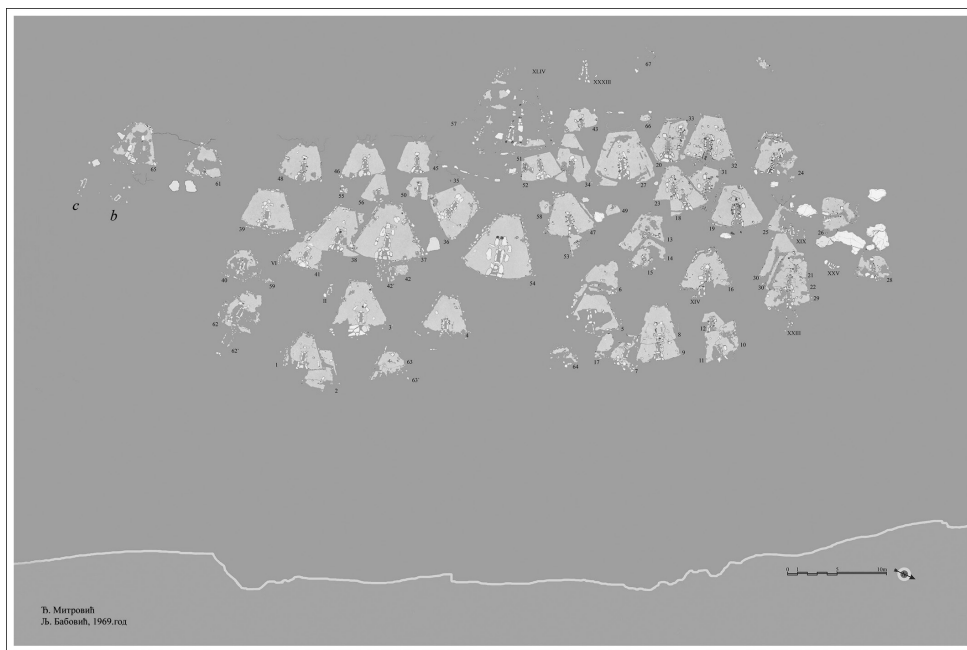
Слика 3. Ситуациони план светилишта Л.В. I из 1969.год.
