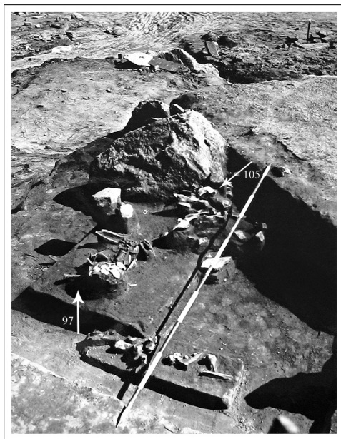
Слика 63. Св. 31, Јесења равноднев., гр. 97,105
