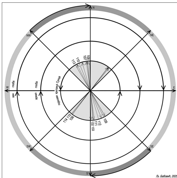
Слика 43. Оријентације скелета новорођенчади, у сфери дана
