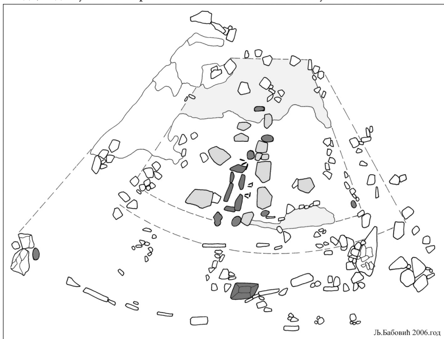
Слика 77. Основа св. XLIV, Хијерогамија богова
