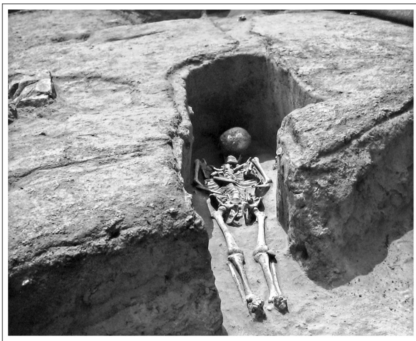
Слика 73. Св. 34, гр. 26
