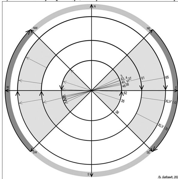
Слика 45. Оријентације свет. са сахрањима, у сфери дана
