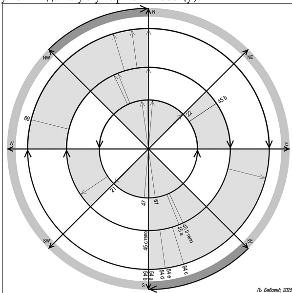
Слика 44. Оријентације скелета осталих узраста у сфери дана
