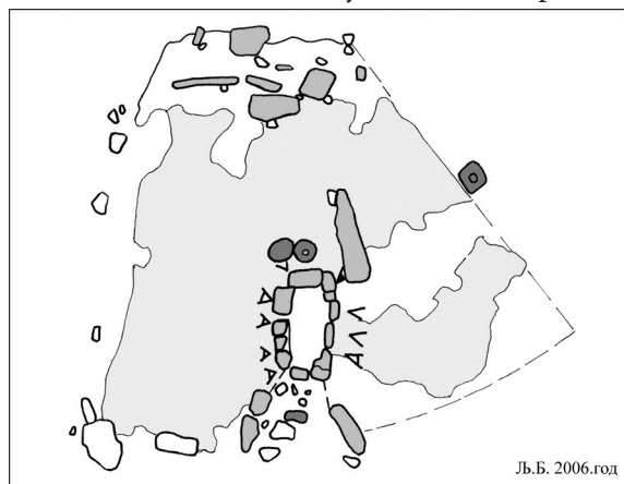
Слика 48а. Основа св. 24, Св. Пуног Месеца
