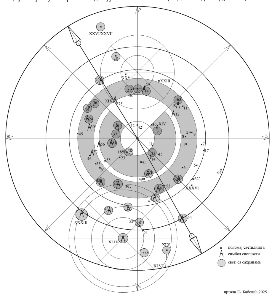
Слика 85. Положај свет. са сахрањима полусфера дана и ноћи, у оквиру глоба
