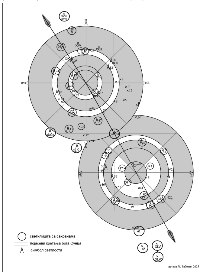
Слика 5. План свет. полусфера дана и ноћи, у односу на осу сфера, са означеним свет. са сахранама
