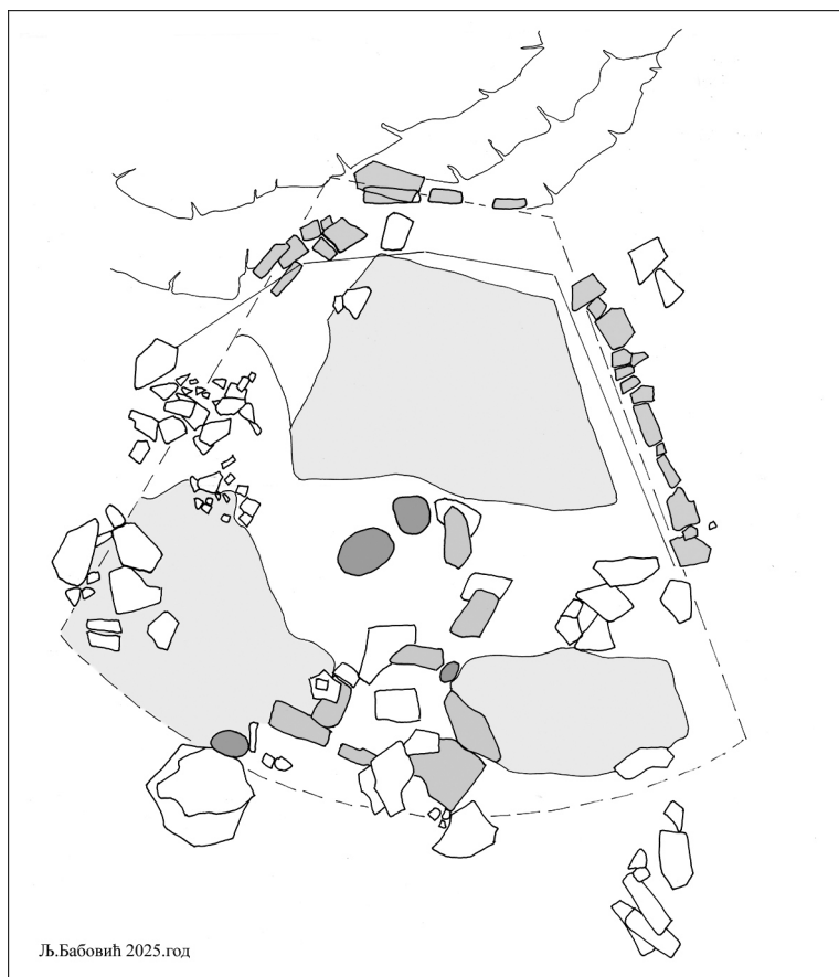
Слика 20. Основа св. 61 и кам. кон. XXXIV, Јужни Сунчев Обрт
