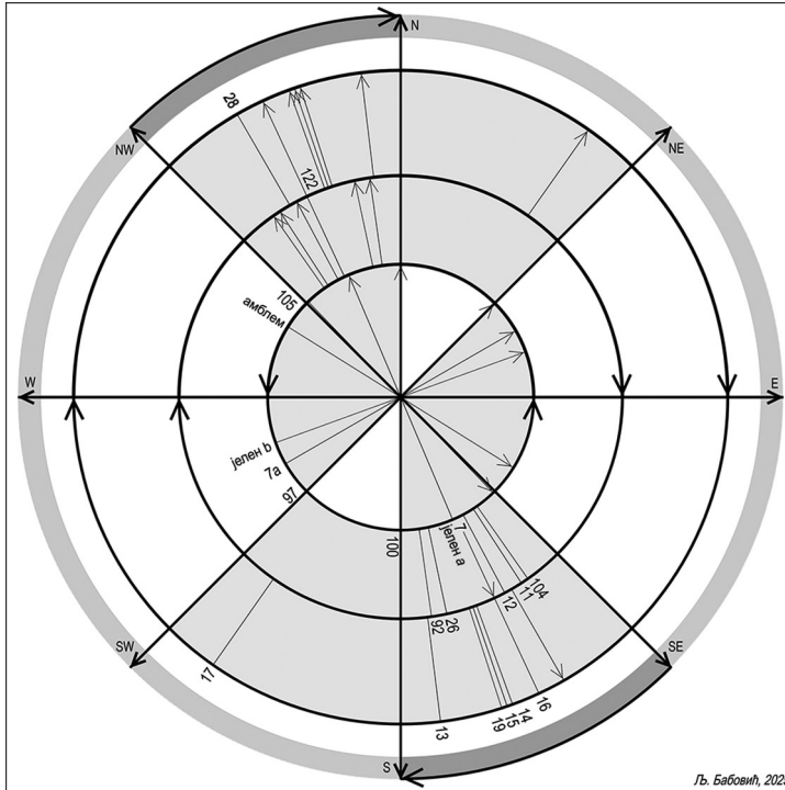
Слика 83. Оријентације скелета осталих узраста, у сфери ноћи
