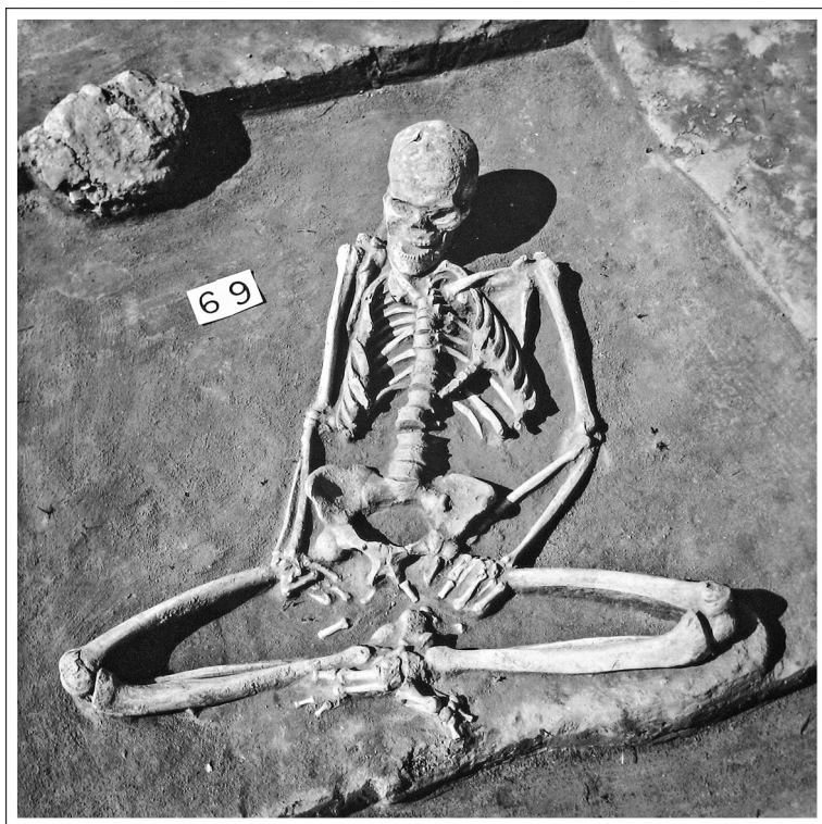
Слика 40. Св. XLV Сунчева палата; гр. 69 у лотос положају, са И
