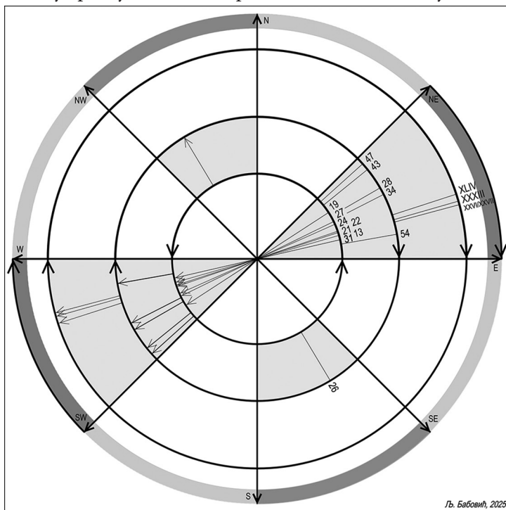
Слика 84. Оријентације свет. са сахранама, у сфери ноћи
