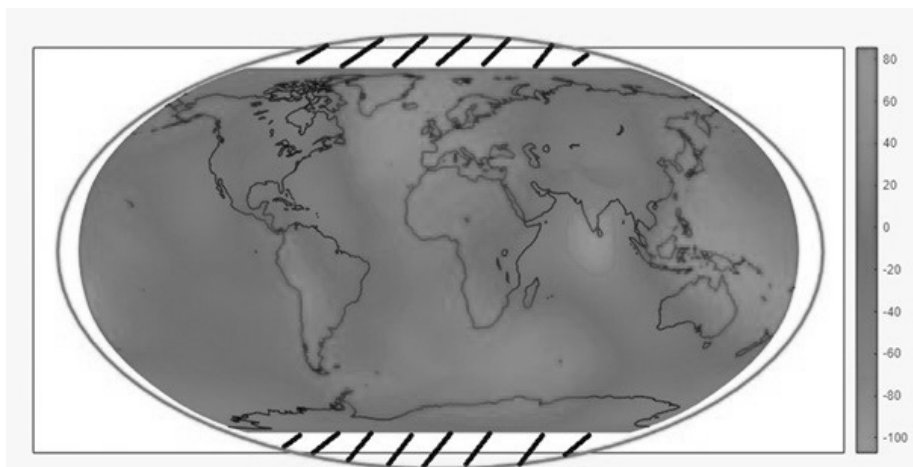
Слика 2. Простор Земљине кугле, на ком надметање гравитационе силе, центрипеталне силе, и силе аеродинамичког отпора одређује латитуду пада метеорита. Слика је направљена у програму Матлаб (MathWorks Inc, 2022).
